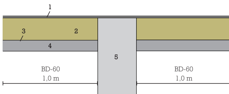
Figur 15: Brandkammerstatning
