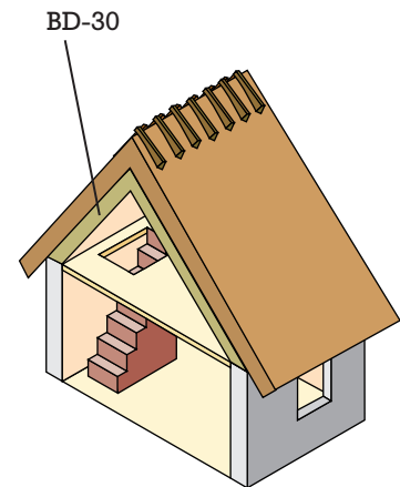
Figur 10b: Beboet tagrum BD-30 konstruktion under stråtag
