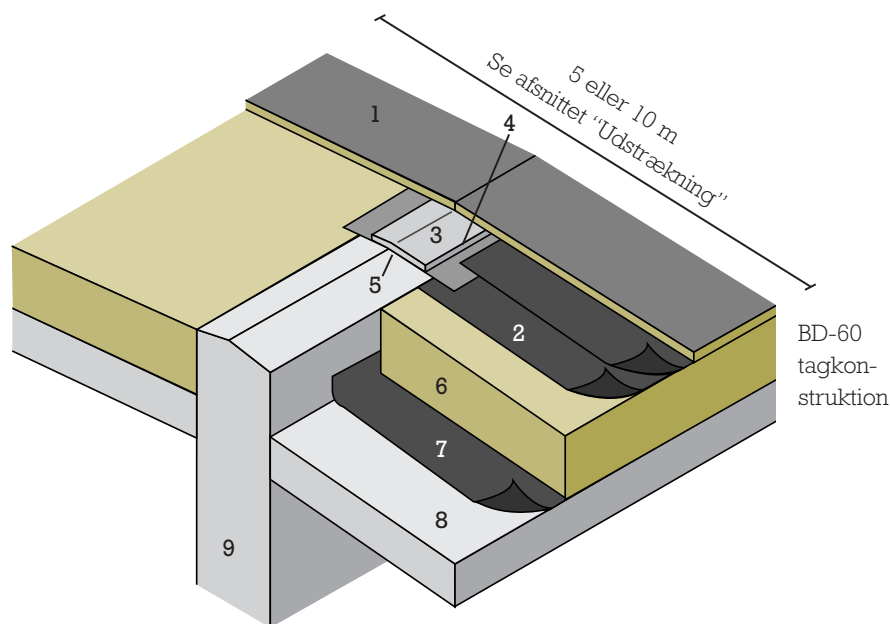
Figur 17: Brandkamserstatning. Den samlede tagkonstruktion skal opbygges som BD-60 tagkonstruktion.
