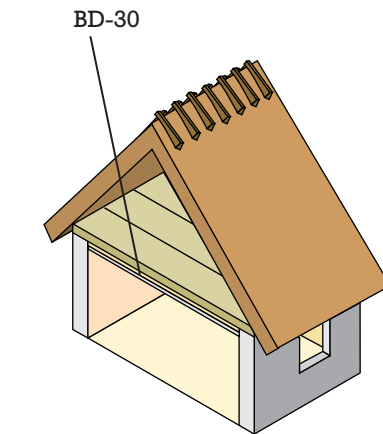
Figur 10a: Udnyttet tagrum Brandsikring anbefales, men ikke lovkrav Etageadskillelse BD-30, se figur 19.
