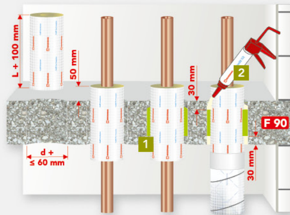
1 Steinwolle-Stopfung, 120 kg/m³ 2 Conlit Kit
