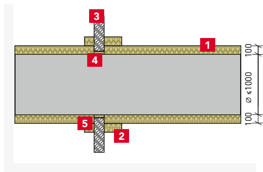
4.3 b att. Ventilācijas gaisa kanāla, kas izolēts ar CONLIT MAT ruļļpaklājiem, izvadīšana cauri betona vai mūra sienai:
