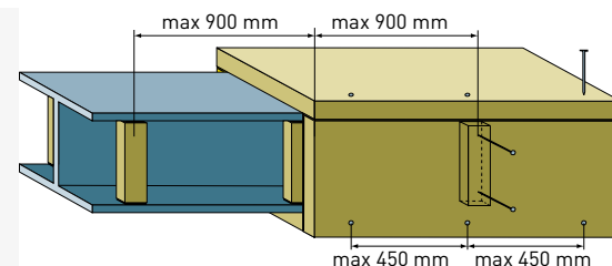
1.2 att. Tērauda sijas, kad tās augstums h < 500\text{ mm} , aizsardzība pret uguni izmantojot CONLIT 150 sistēmu
