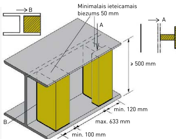
1.3 att. Tērauda sijas, kad tās augstums h \geq 500\text{ mm} , aizsardzība pret uguni izmantojot CONLIT 150 sistēmu
