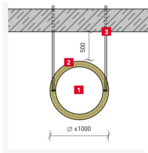
4.2 att. Ventilācijas gaisa kanālu piekarināšana – griezumā pie piekarināšanas ietaišēm
