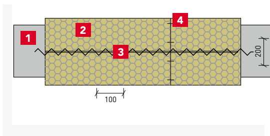
4.1 att. Stieples sieta sastiprināšana:
