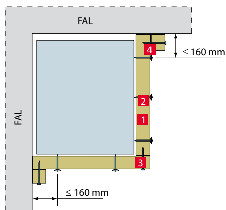
CONLIT Ductrock / Plus lemezekkel kétoldalúan szigetelt függőleges csatorna
