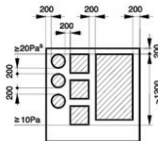
Een combinatie van enkelvoudige leidingen. Tussen elke sparing zit minimaal 200 mm afstand.
