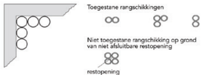
Testopstelling van leidingen naast en boven elkaar. Rechts de rangschikkingen die op grond hiervan zijn toegestaan. De vierkantvorm is niet toegestaan.
