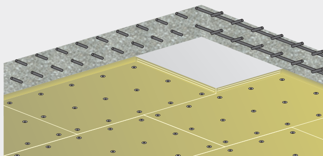
Étape 1 : excellentes propriétés antifeu grâce à Conlit Steelprotect Board
