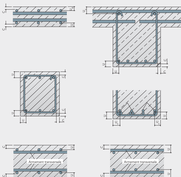
Illu. 3 : Distances u , u_o et u_s ainsi qu'épaisseur de recouvrement c
