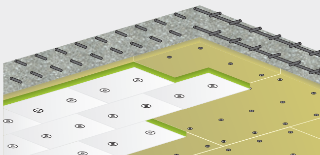
Étape 2 : isolation thermique très efficace grâce à un panneau isolant ROCKWOOL supplémentaire
