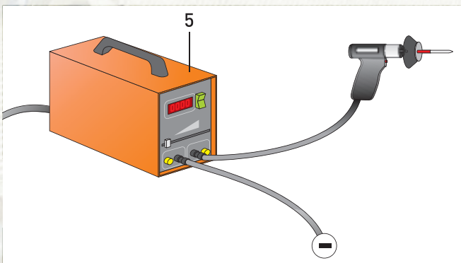
Appareil à souder Pin-Spot et chevilles à souder
