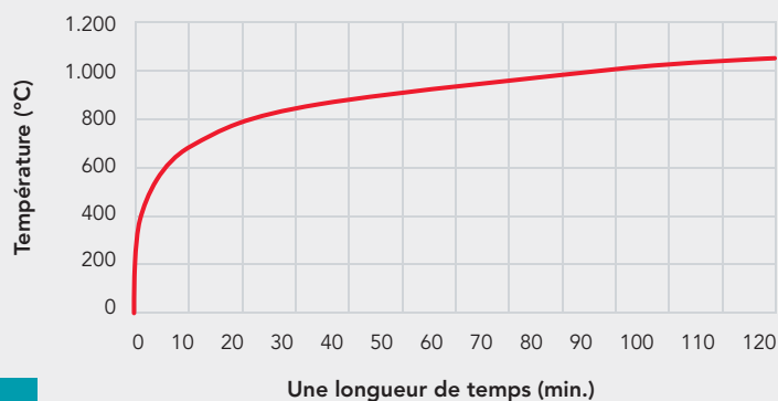
La courbe ISO 834
