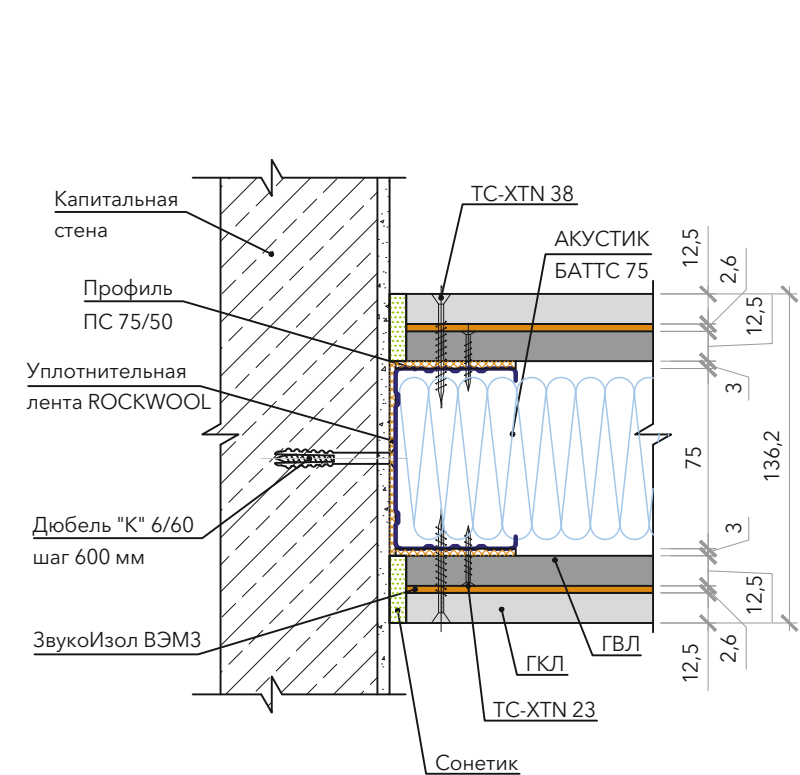
Примыкание перегородки к капитальной стене
