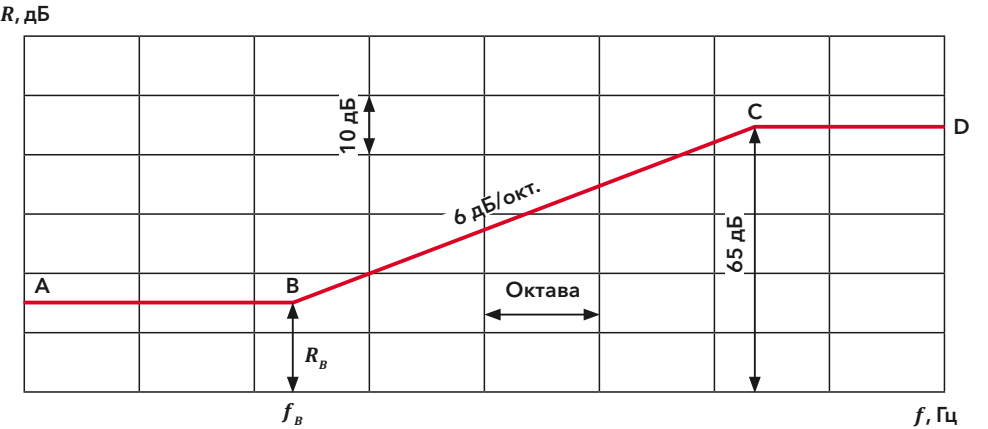
Рисунок 1. Частотная характеристика изоляции воздушного шума однослойным плоским ограждением
