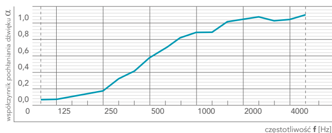
TECHROCK 80 FB1, grub. 20 mm, z jednostronną okładziną z welonu szklanego
