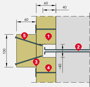
Sposób izolacji w miejscach połączeń kołnierowych o wysokości większej niż 30 mm
