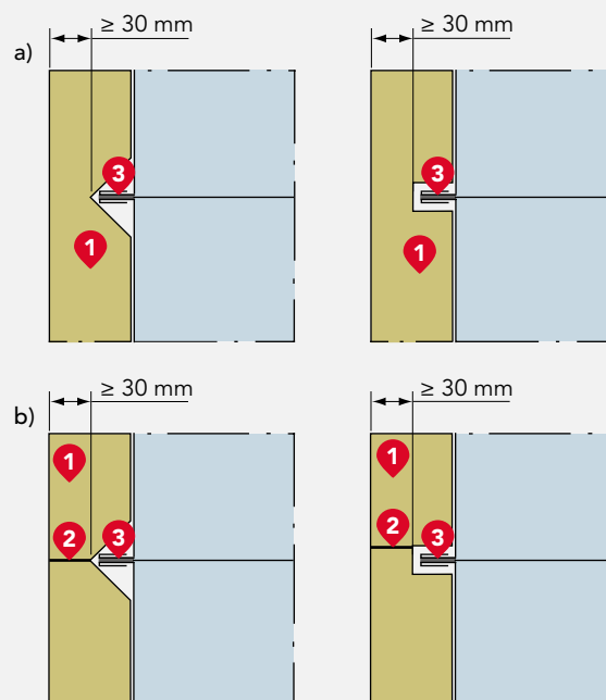
Sposób izolacji połączeń kołnierowych
