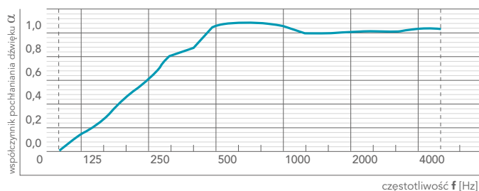
TECHROCK 60 FB1, grub. 50 mm, z jednostronną okładziną z welonu szklanego
