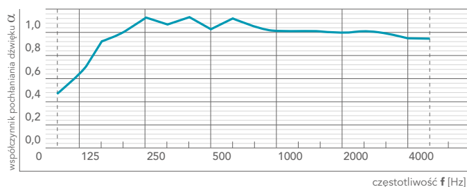
TECHROCK 60 FB2, grub. 100 mm, z dwustronną okładziną z welonu szklanego
