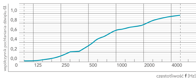
TECHROCK 80 FB1, grub. 15 mm, z jednostronną okładziną z welonu szklanego
