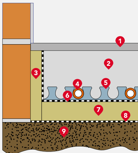
1. Warstwa wykończeniowa, 2. Podkład cementowy, 3. Pasek RST, 4. Rura ogrzewania, 5. Mata montażowa, 6. Folia paroizolacyjna, 7. Płyta z wełny STEPROCK BASE , 8. Izolacja przeciwwilgociowa lub przeciwwodna, wg potrzeb, 9. Grunt/strop.
