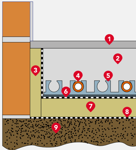
1. Warstwa wykończeniowa, 2. Podkład cementowy, 3. Pas RST, 4. Przewód ogrzewania płaszczyznowego, 5. Szyna montażowa, 6. Folia paroizolacyjna, 7. Płyta z wełny STEPROCK BASE , 8. Izolacja przeciwwilgociowa lub przeciwwodna, wg potrzeb, 9. Grunt/strop.
