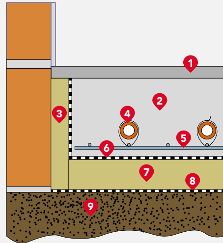
1. Warstwa wykończeniowa, 2. Podkład cementowy, 3. Pas RST, 4. Rura ogrzewania, 5. Siatka montażowa/zbrojeniowa, 6. Folia paroizolacyjna, 7. Płyta z wełny STEPROCK BASE , 8. Izolacja przeciwwilgociowa lub przeciwwodna, wg potrzeb, 9. Grunt/strop.
