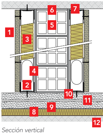
Sección vertical
