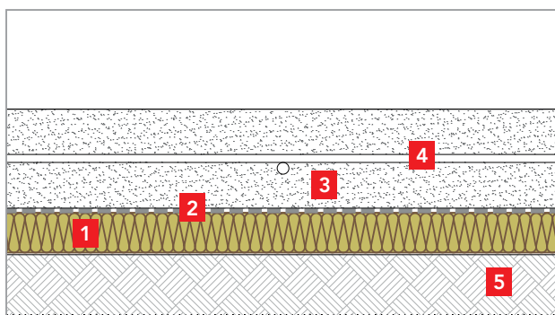
Sección vertical
