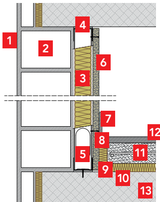
Sección vertical
