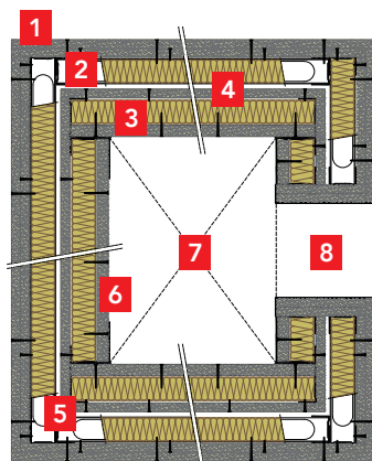
Secção em planta
