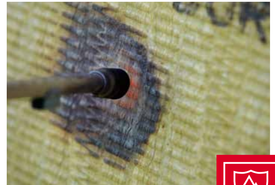
Steinwolle im Brandversuch
