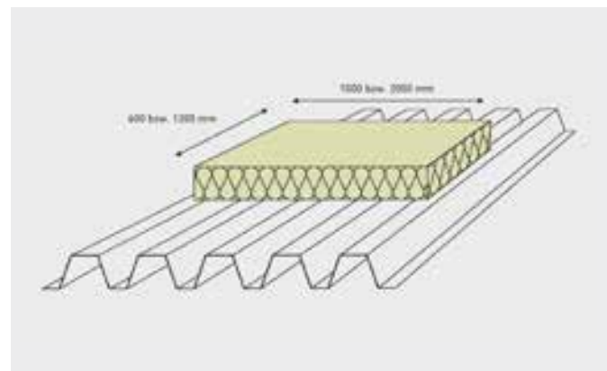
Verlegerichtung auf Trapezprofildächern
