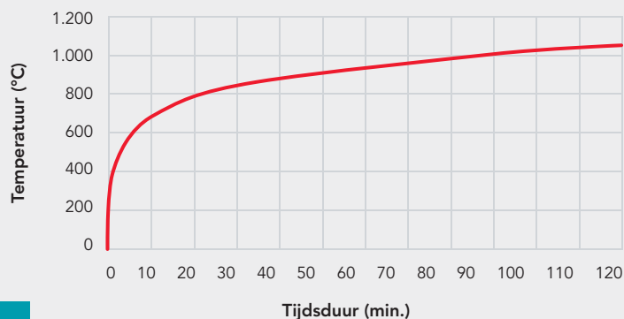
ISO 834 brandkromme
