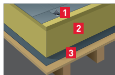
Figur 41: Varmt tag på trækonstruktion
