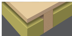
Figur 5: Ventilationsspalte på ca. 7 - 8 cm
