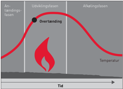
Figur 12: viser et standard brandforløb fra antænding til overtænding og afkøling. Ved anvendelse af brændbar isolering forskydes kurven mod venstre, hvorved overtænding kan forventes meget hurtigt efter antænding.
