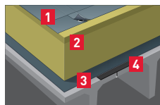
Figur 42: Varmt tag på betonelementdæk
