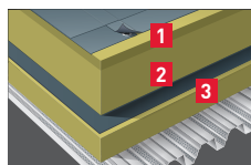
Figur 40: Varmt tag på ståltrapez
