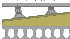
Figur 25: HARDKILE Eksempel på opbygning
