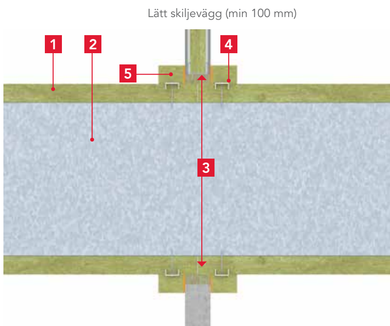
Massiv vägg (min 100 mm)
