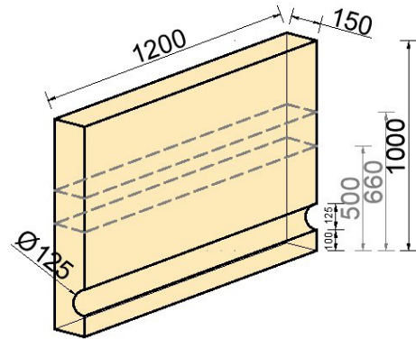
Figuur 1: Rockflow element uitvoeringen
