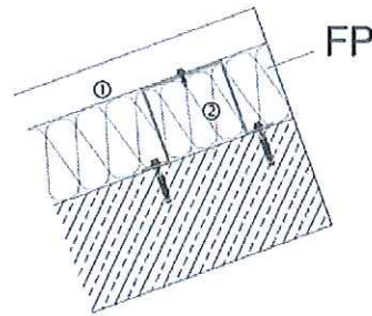
Unterkonstruktion: Beton oder Porenbeton Festpunkt (FP): Kantenteil aus Stahl o.a.
