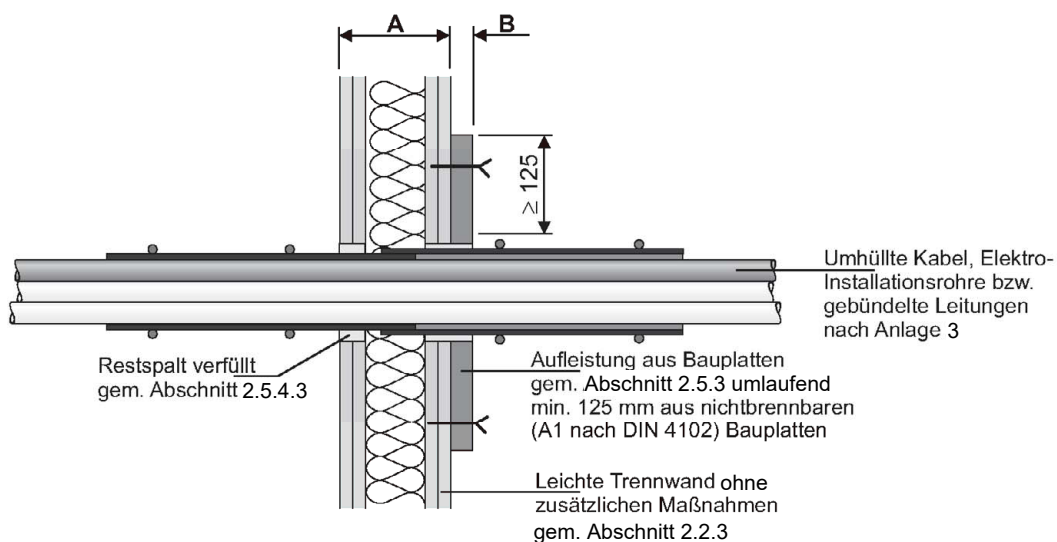
Mindestbauteildicke und Aufleistung für Massivwände
